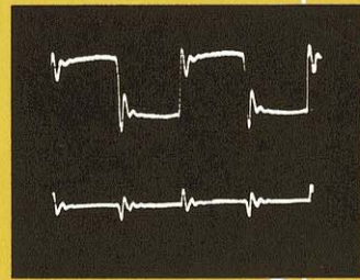
Rechteckwiedergabe: oben Summe aus rechtem und linkem Kanal, unten Differenz
